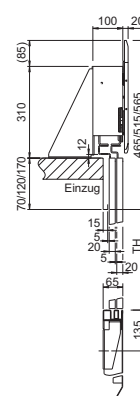
schmale Kabinentür e2
