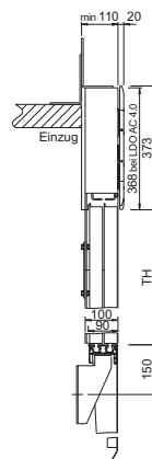
Kabinentür MOD m4
