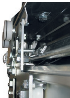
Verstärkte Fahrschlitten mit Rückhalteeinrichtung an der Sicherungsschiene
