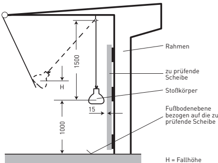
Pendelschlagversuch Anforderungen vollständig erfüllt
