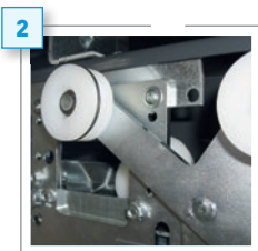
Rückhalteeinrichtung am Fahrschlitten zum Kämpfen bei Versagen der oberen Führung
