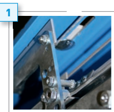
Verstärkte Fahrschlitten mit Rückhalteeinrichtung an der Sicherungsschiene
